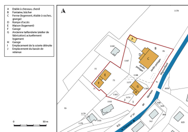
Plan-masse et de situation. Extrait du plan cadastral, 2017, section B, 1/2 500 agrandi à 1/1 000. Dess. Bertrand Turina IVR43_20182501317NUDA
