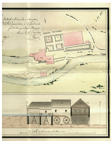
Plan et profil relatifs à la demande en autorisation d'usine formée par le Sr Joseph Bobillier, propriétaire à la Grand'Combe [détail], 15 juillet 1822. Phot. Jérôme Mongreville, Autr. Vauquelin IVR43_20182500030NUC4A
