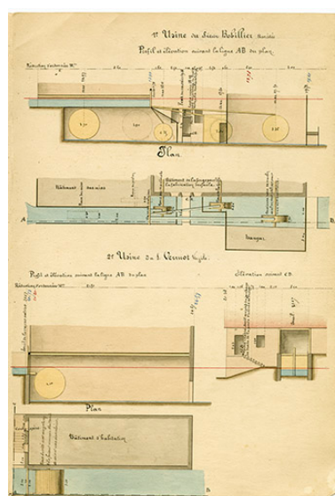
Commune de Grand'Combe. Règlement d'eau des usines [...] Dessins de détails [usines Bobillier et Vermot], 21 juin 1876. Autr. Couturier IVR43_20182500031NUC4A
