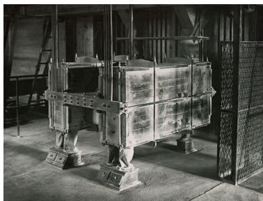
Plansichter, s.d. [vers 1960]. IVR43_20192500068NUC4A
