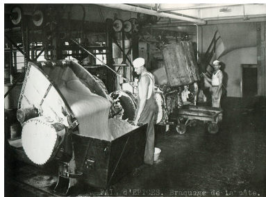
Atelier des pains d'épices. Braquage de la pâte, s.d. [vers 1960]. IVR43_20192500080NUC2A
