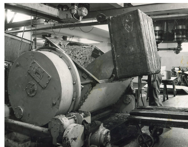
Atelier des pains d'épices. Versement de la pâte (?), s.d. [vers 1960]. IVR43_20192500075NUC4A
