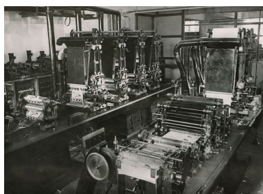
Atelier d'imprimerie, s.d. [vers 1960]. IVR43_20192500067NUC4A
