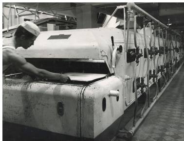
Atelier des pains d'épices. Four continu, s.d. [vers 1960]. IVR43_20192500076NUC4A
