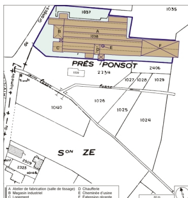
Plan-masse et de situation. Extrait du plan cadastral numérisé, 2006, section A, 1:1250 agrandi à 1:1000. Dess. André Céréza IVR43_20067000069NUDA
