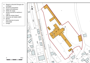
Plan-masse et de situation. Extrait du plan cadastral, 2015, section AE. Dess. Mathias Papigny IVR43_20162500942NUDA
