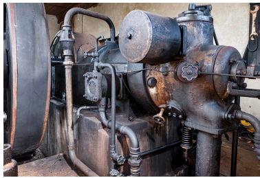
Moteur diesel Duvant. Détail. Phot. Jérôme Mongreville IVR43_20152502400NUC4A
