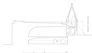
Boulevard dit Grosse Tour. Coupe A-A'.
