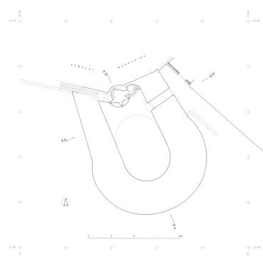
Boulevard dit Grosse Tour. Plan niveau supérieur.
