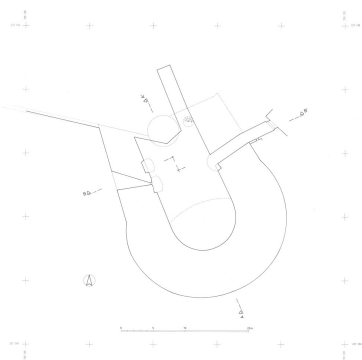
Boulevard dit Grosse Tour. Plan niveau inférieur.
