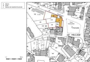
Plan de masse et de situation. Dess. Mathias Papigny IVR43_20157001491NUDA
