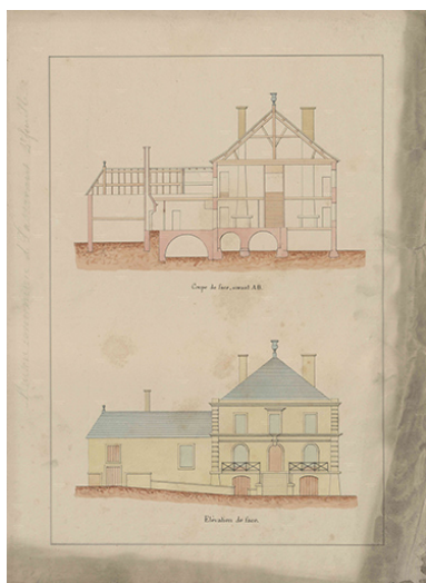
Plan présentant l'élévation et la coupe de face de la façade antérieure. Autr. auteur inconnu IVR43_20167000059NUC4A
