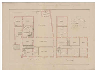
Plan du rez-de-chaussée et du 1er étage (fin 19e siècle). Autr. auteur inconnu IVR43_20167000058NUC4A
