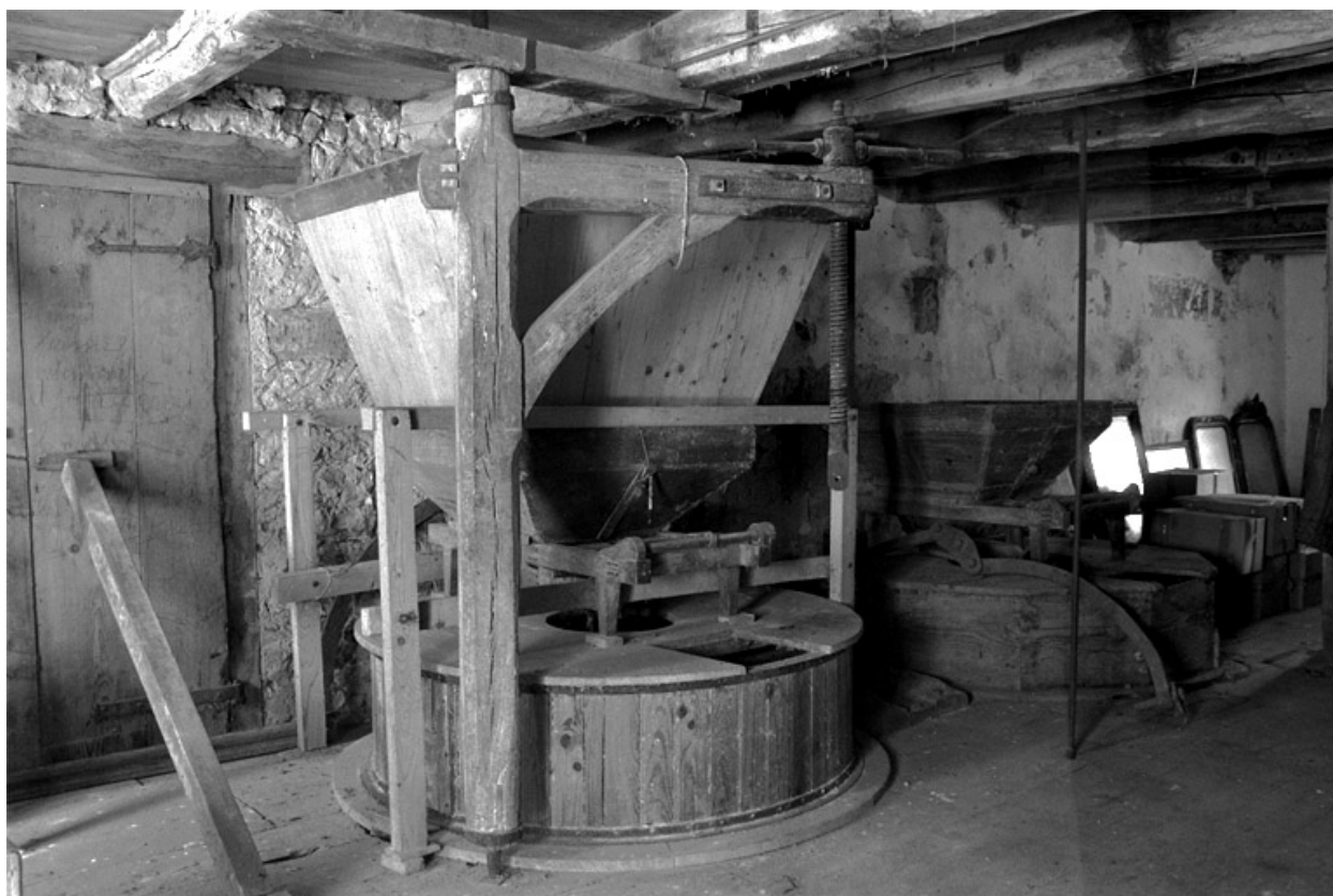
Meules (étage carré).
