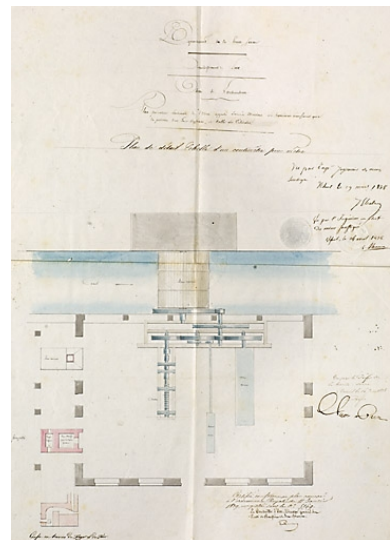
Plan présentant l'ensemble de l'usine appelée ancien martinets au laminoir neuf ainsi que la position d'un four d'affinerie, et celle du cylindre. Phot. Jérôme Mongreville IVR43_20077000071NUCA
