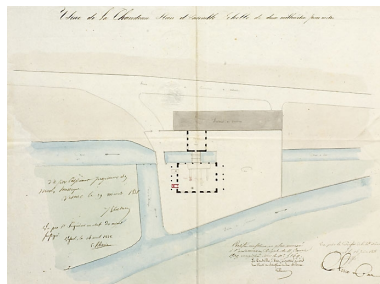
Usine de la Chaudeau. Plan d'ensemble. Phot. Jérôme Mongreville IVR43_20077000072NUCA
