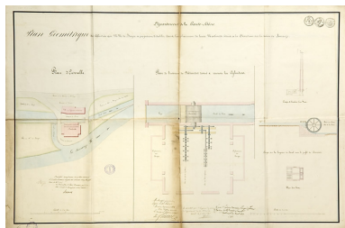
Plan géométrique des cylindres que MM. de Buyer se proposent d'établir dans l'emplacement de leurs martinets [...]. Phot. Jérôme Mongreville IVR43_20077000070NUCA
