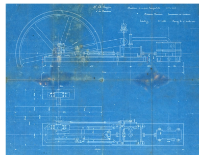
Machine à vapeur horizontale Farcot. Phot. Jérôme Mongreville IVR43_20077000062NUCA
