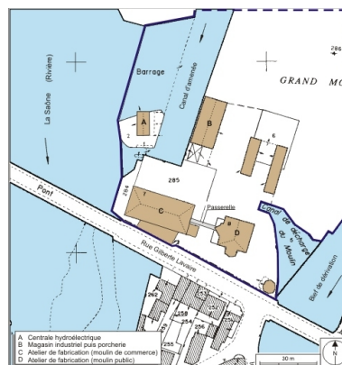
Plan-masse et de situation. Extrait du plan cadastral numérisé, 2008, section BT, 1:1000. Source : Direction générale des Finances Publiques - Cadastre ; mise à jour : 2008. Dess. André Céréza IVR43_20087000500NUDA
