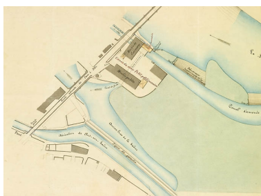
Plan des lieux [Plan-masse et de situation]. Phot. Jérôme Mongreville, Autr. Becker IVR43_20097000042NUC2A
