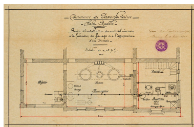
Chalet-modèle. Projet d'installation du matériel nécessaire à la fabrication des fromages et à l'appropriation d'une beurrerie, 1910. Phot. Jérôme Mongreville IVR43_20152500585NUC4A
