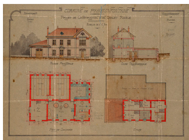
Commune de Passonfontaine. Projet de construction d'un chalet-modèle, 1910. Phot. Jérôme Mongreville IVR43_20152500583NUC4A
