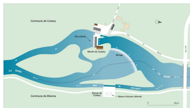
Plan schématique du site de l'écluse de Cuisery, du barrage et du moulin. Dess. Alain Morelière IVR26_20137100003NUDA
