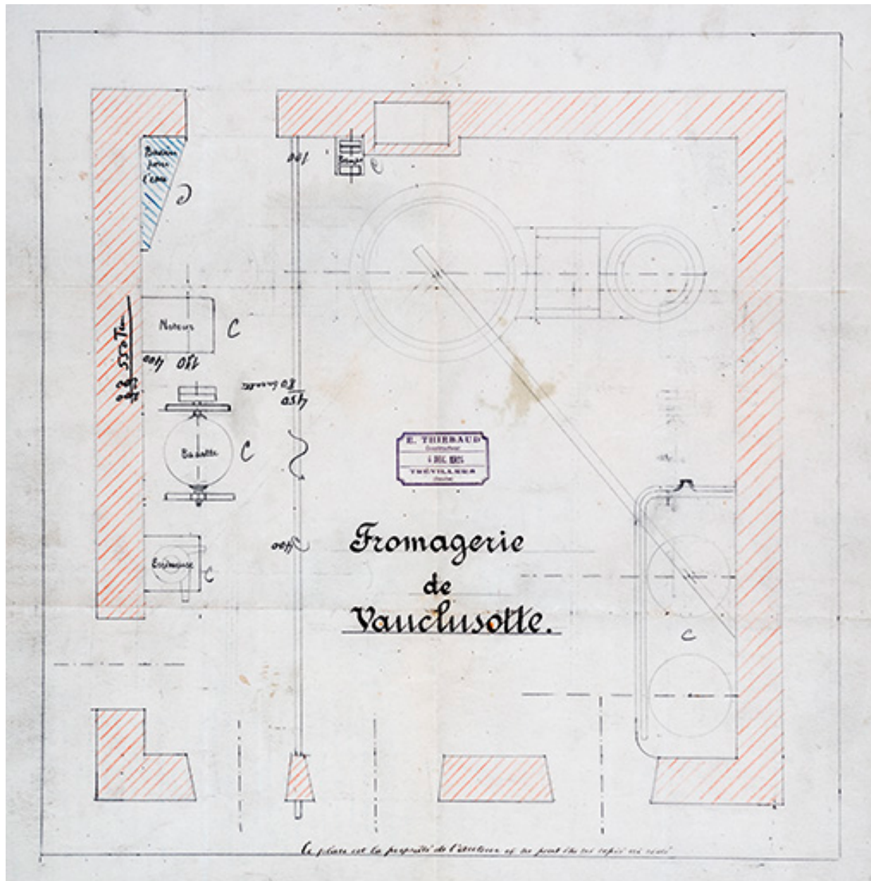
Fromagerie de Vaclusotte [schéma d'implantation de l'équipement], 1924.
