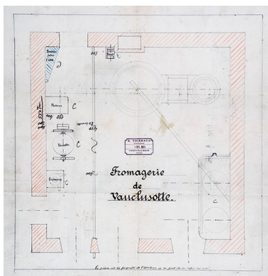
Fromagerie de Vaclusotte [schéma d'implantation de l'équipement], 1924. Phot. Jérôme Mongreville, Autr. Ets Emile Thiébaud IVR43_20152500563NUC4A
