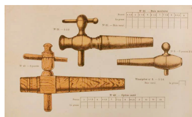
Articles de tournerie vendu vendu par la société dans les années 1920 : robinets. Phot. Jérôme Mongreville IVR43_19923900303XA
