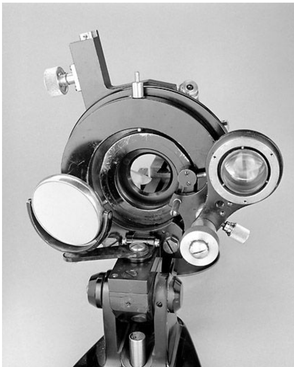
Troisième microscope : face inférieure de la platine.
