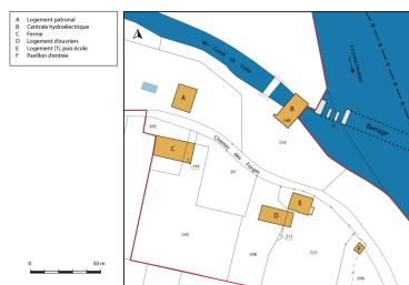
Plan-masse et de situation. Extrait du plan cadastral, 2019. Dess. Bertrand Turina IVR43_20192501049NUDA
