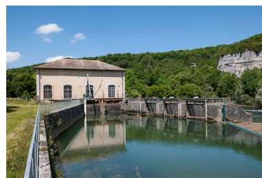
La centrale vue depuis la rive droite du barrage. Phot. Jérôme Mongreville IVR43_20152501205NUC4A
