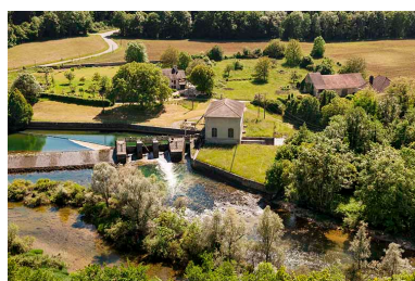
Vue plongeante depuis le nord-est. Phot. Jérôme Mongreville IVR43_20152501224NUC4A
