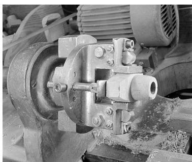
Mandrin "gueule de loup" (atelier de finissage). Phot. Jérôme Mongreville
