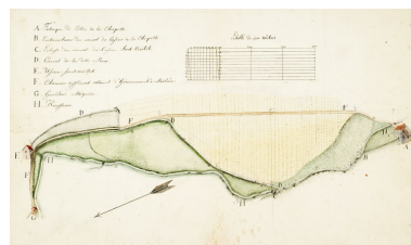
Usine Peugeot Frères [Plan de situation des usines Sous- Cratet et de la Chapotte]. Papier, plume, lavis, s.d. [vers 1810]. Phot. Jérôme Mongreville IVR43_20112500308NUC4A
