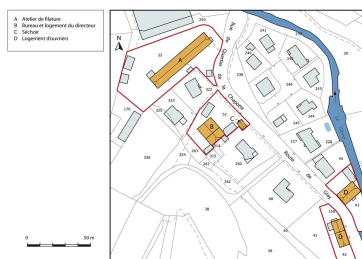
Plan-masse et de situation. Dess. Mathias Papigny IVR43_20132502625NUDA
