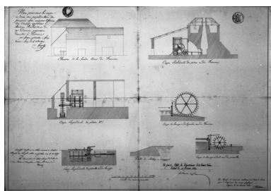
Plan présentant la coupe en deux sens perpendiculaires des principaux objets composant le fourneau du Crochot [...]. Phot. Yves Sancey, Phot. Guyet IVR43_19877000059X
