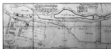
Plan de l'usine du Crochot [...].
