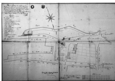
Plan de l'usine du Crochot composée d'un haut fourneau avec soufflerie à pistons, d'un patouillet, de bâtiments servant à son exploitation [...]. Phot. Yves Sancey, Phot. Guyet IVR43_19877000061X
