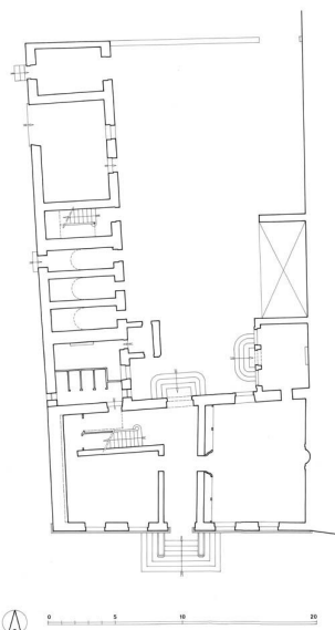
Plan du rez-de-chaussée. Dess. Alain Morelière IVR26_20122100832A2YY
