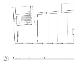
Plan de l'étage. Dess. Alain Morelière IVR26_20122100834A2YY
