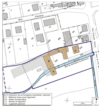
Plan-masse et de situation. Extrait du plan cadastral numérisé, 2008, section AT, 1:1000. Source : Direction générale des Finances Publiques - Cadastre ; mise à jour : 2008. Dess. André Céréza IVR43_20087000351NUDA
