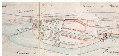
Usine de Bourguignon et dépendances, plan des lieux et des ouvrages projetés, [détail], tirage, échelle 1/1000, le 17/07/1920.
