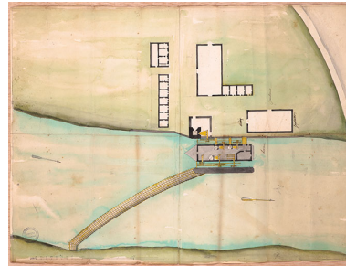
Plan des forges appartenantes à Mgr le maréchal duc de Lorges et à Mme la maréchale duchesse de Lorges son épouse [...], levé par Gallezot, géomètre, plume, lavis, s.d. [1744] Phot. Jérôme Mongreville IVR43_20132500517NUC4A
