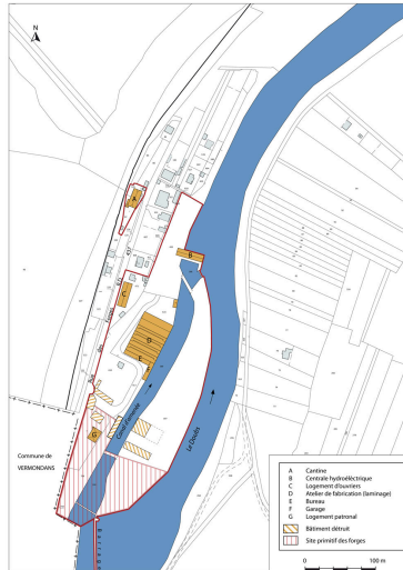
Plan-masse et de situation. Extrait du plan cadastral numérisé, section D, échelle 1:2000. Dess. Mathias Papigny IVR43_20142500575NUDA
