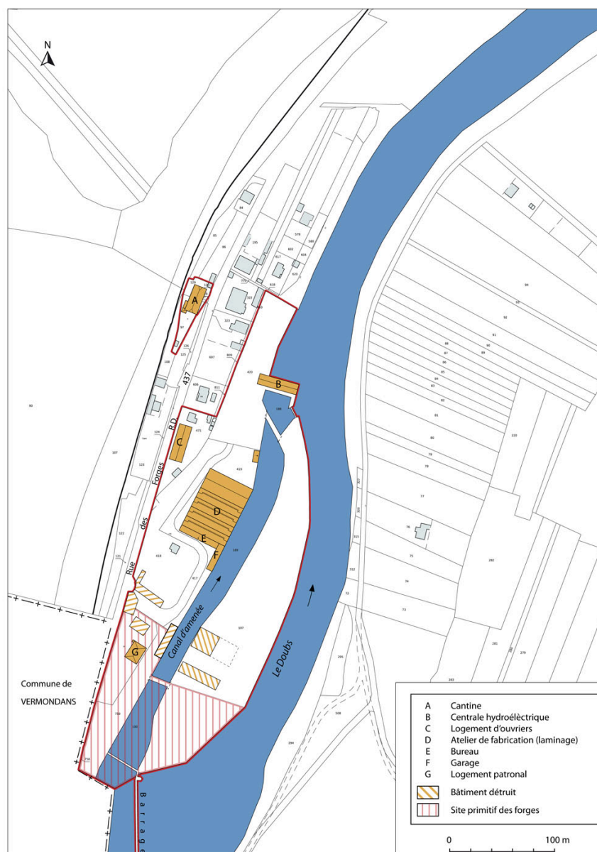
Plan-masse et de situation. Extrait du plan cadastral numérisé, section D, échelle 1:2000.
