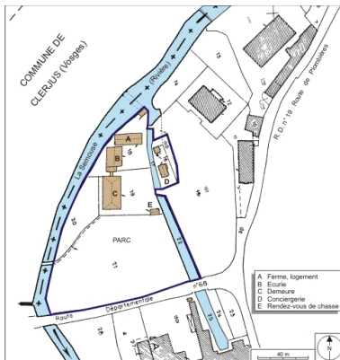
Plan-masse et de situation. Extrait du plan cadastral numérisé, 2008, section A, 1:1250 réduit à 1:1500. Source : Direction générale des Finances Publiques - Cadastre ; mise à jour : 2008. Dess. André Céréza IVR43_20087000228NUDA
