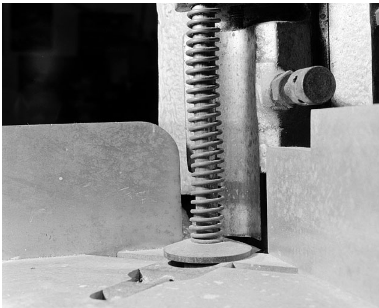
Détail du presse-papiers et du tranchoir.
