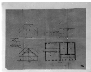
Projet de construction d'une cuisine et d'une laiterie pour le chalet [plan, coupe et élévations]. Phot. Yves Sancey, Phot. Narcisse Perrard IVR43_19973901968V
