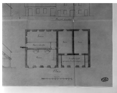
Projet de construction d'une cuisine [...] Plan. Phot. Yves Sancey, Phot. Narcisse Perrard IVR43_19973901969V
