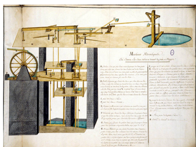
Machines Hydrauliques Qui Elèvent Les Eaux salées et douces du puits à Muire [partie droite], 1756. Phot. Yves Sancey, Autr. Dorval IVR43_19943900215ZA
