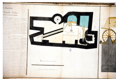
Machines Hydrauliques Qui Elèvent Les Eaux salées et douces du puits à Muire [plan du puits à muire], 1756. Phot. Yves Sancey, Autr. Dorval IVR43_19943900212ZA
