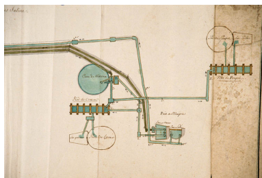
Plan des différents cours des eaux salées et douces des grande et petites salines de Salins [détail de la petite saline], 1756. Phot. Yves Sancey, Autr. Dorval IVR43_19943900184ZA
