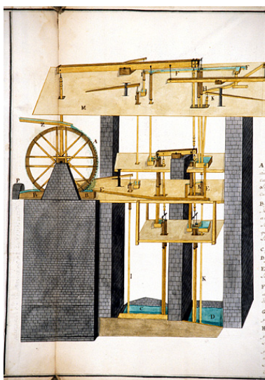
Machines Hydrauliques Qui Elèvent Les Eaux salées et douces du puits à Muire [détail du système d'élévation], 1756. Phot. Yves Sancey, Autr. Dorval IVR43_19943900218ZA
