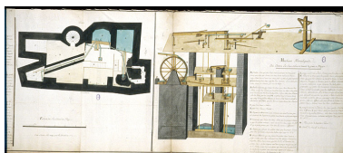
Machines Hydrauliques Qui Elèvent Les Eaux salées et douces du puits à Muire, 1756. Phot. Yves Sancey, Autr. Dorval IVR43_19943900209ZA
