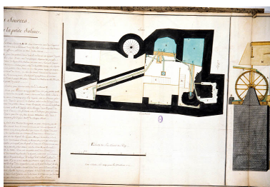
Machines Hydrauliques Qui Elèvent Les Eaux salées et douces du puit à Muyre [plan du puits à muire], 1756. Phot. Yves Sancey, Autr. Dorval IVR43_19943900212ZA
