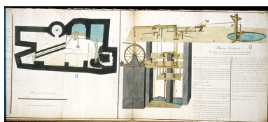
Machines Hydrauliques Qui Elèvent Les Eaux salées et douces du puit à Muyre, 1756. Phot. Yves Sancey, Autr. Dorval IVR43_19943900209ZA
