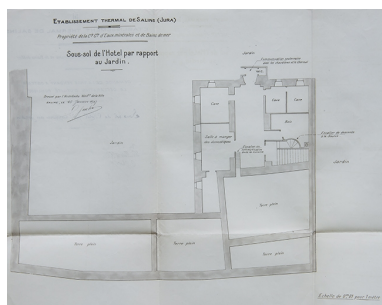
Plan du premier sous-sol (rez-de-jardin) du Grand Hôtel des Bains (1917). Phot. Jérôme Mongreville IVR43_20223900087NUC4A
