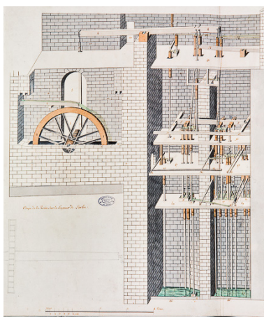
Machine hydraulique pour l'élévation des eaux salées et douces du Puits à muire [... : détail de la partie gauche], s.d. [18e siècle]. Phot. Yves Sancey IVR43_19943900526XA
