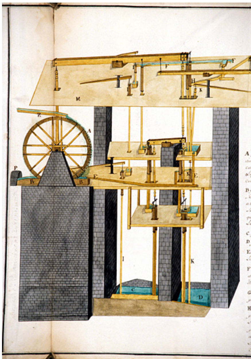
Machines Hydrauliques Qui Elèvent Les Eaux salées et douces du puit à Muyre [détail du système d'élévation], 1756.
