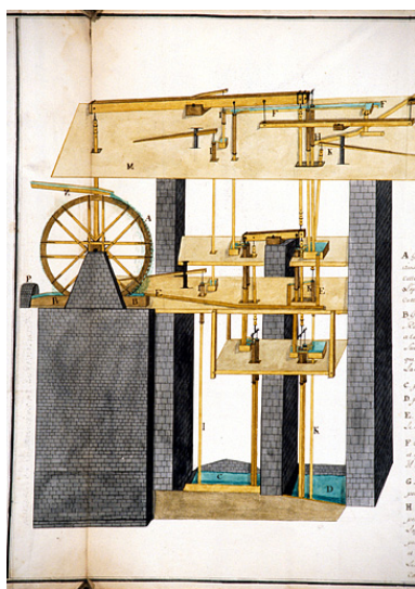
Machines Hydrauliques Qui Elèvent Les Eaux salées et douces du puit à Muyre [détail du système d'élévation], 1756. Phot. Yves Sancey, Autr. Dorval IVR43_19943900218ZA
