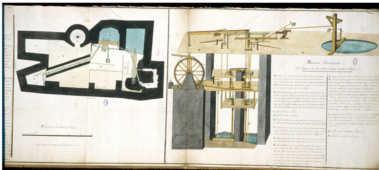
Machines Hydrauliques Qui Elèvent Les Eaux salées et douces du puit à Muyre, 1756.
