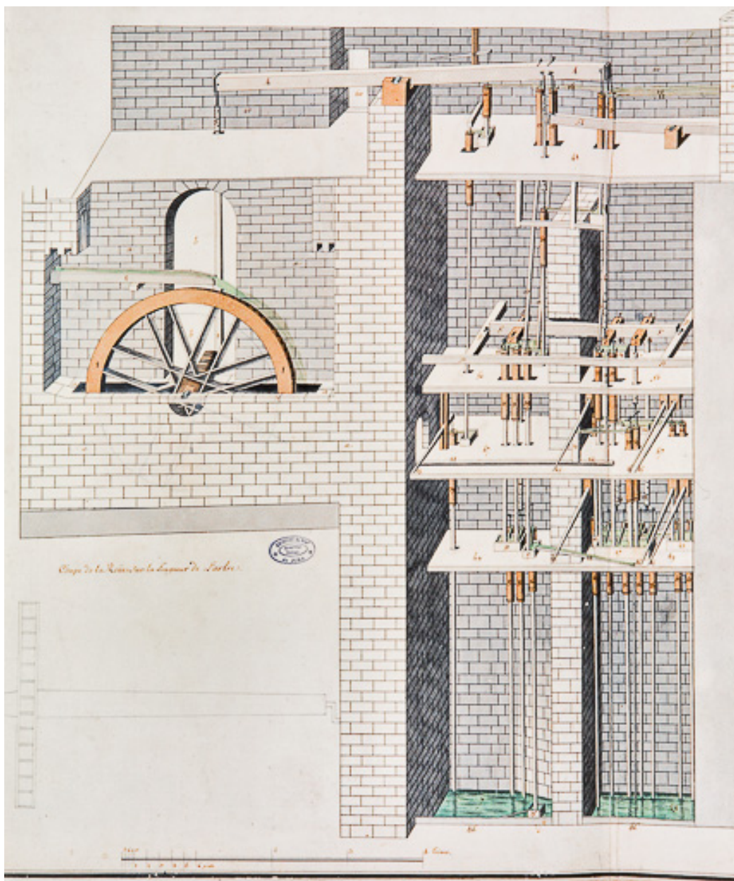
Machine hydraulique pour l'élévation des eaux salées et douces du Puits à muire [... : détail de la partie gauche], s.d. [18e siècle].
