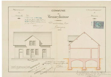
Commune de Vernierfontaine. Construction d'une fromagerie [élévation et coupe transversale], 1881. Phot. Sonia Dourlot IVR43_20152500508NUC4A
