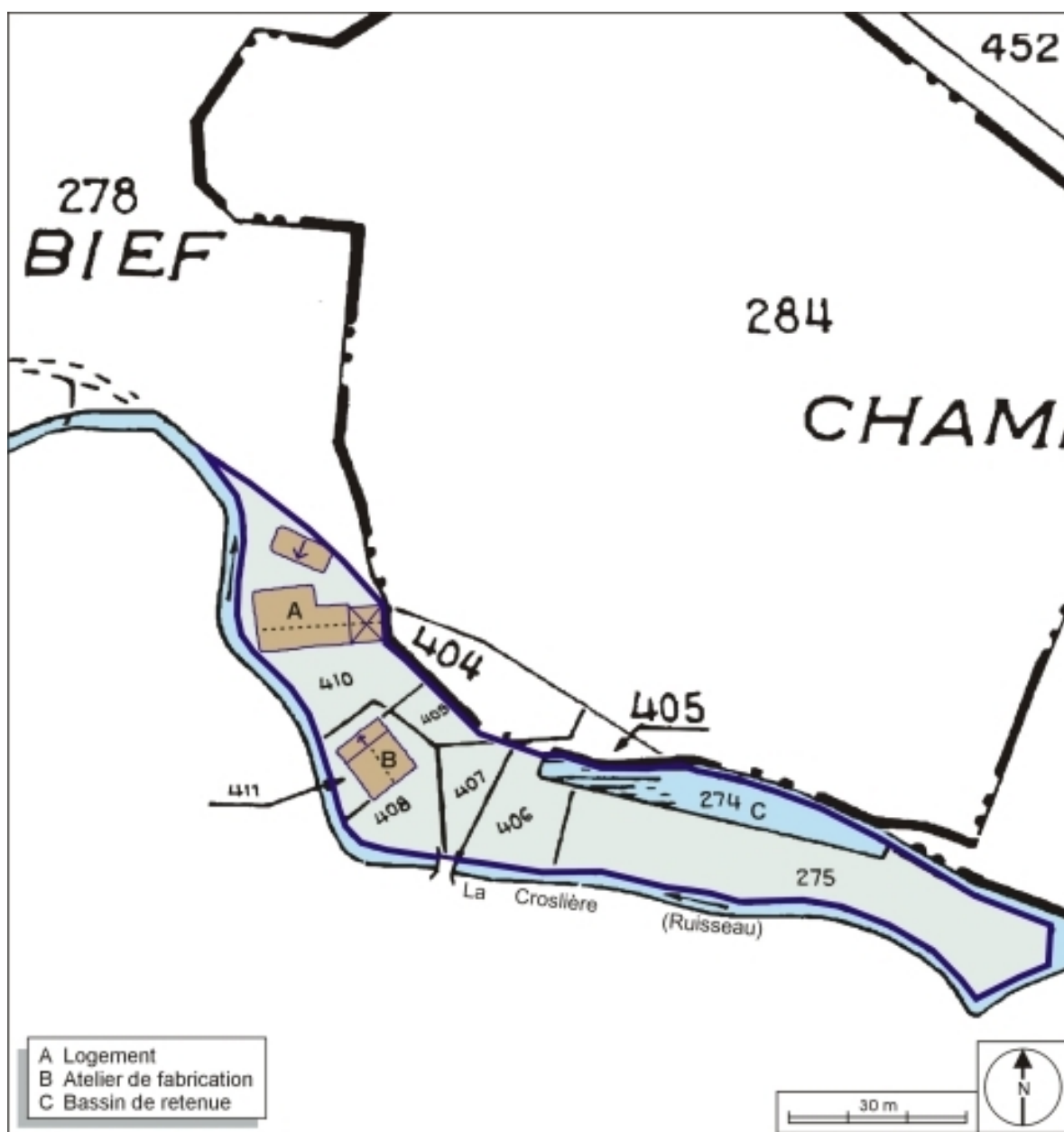
Plan-masse et de situation. Extrait du plan cadastral numérisé, 2005, section B, 1:2500 agrandi à 1:1000.
