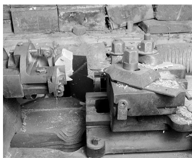
Mandrin gueule de loup et chariot porte-outils. Phot. Jérôme Mongreville IVR43_20003901044X
