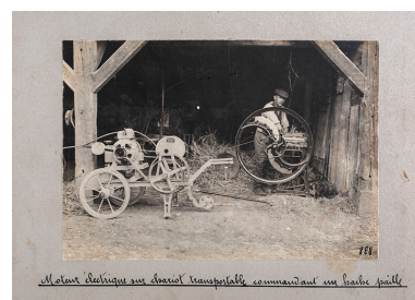
Moteur électrique sur chariot transportable commandant une hache paille, 1ère moitié 20e siècle. Phot. Sonia Dourlot IVR43_20209000060NUC4A
