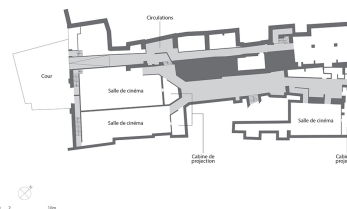
Plan au sous-sol. D'après un plan de la SMCI levé en décembre 2006 par François Gaume et complété en 2018 par le cabinet Coquard, 1/100 réduit à 1/250.
