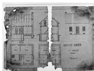
Habitation ouvrière. Cité Chatelot [plan, coupe, élévation]. Phot. Yves Sancey IVR43_19849000005X
