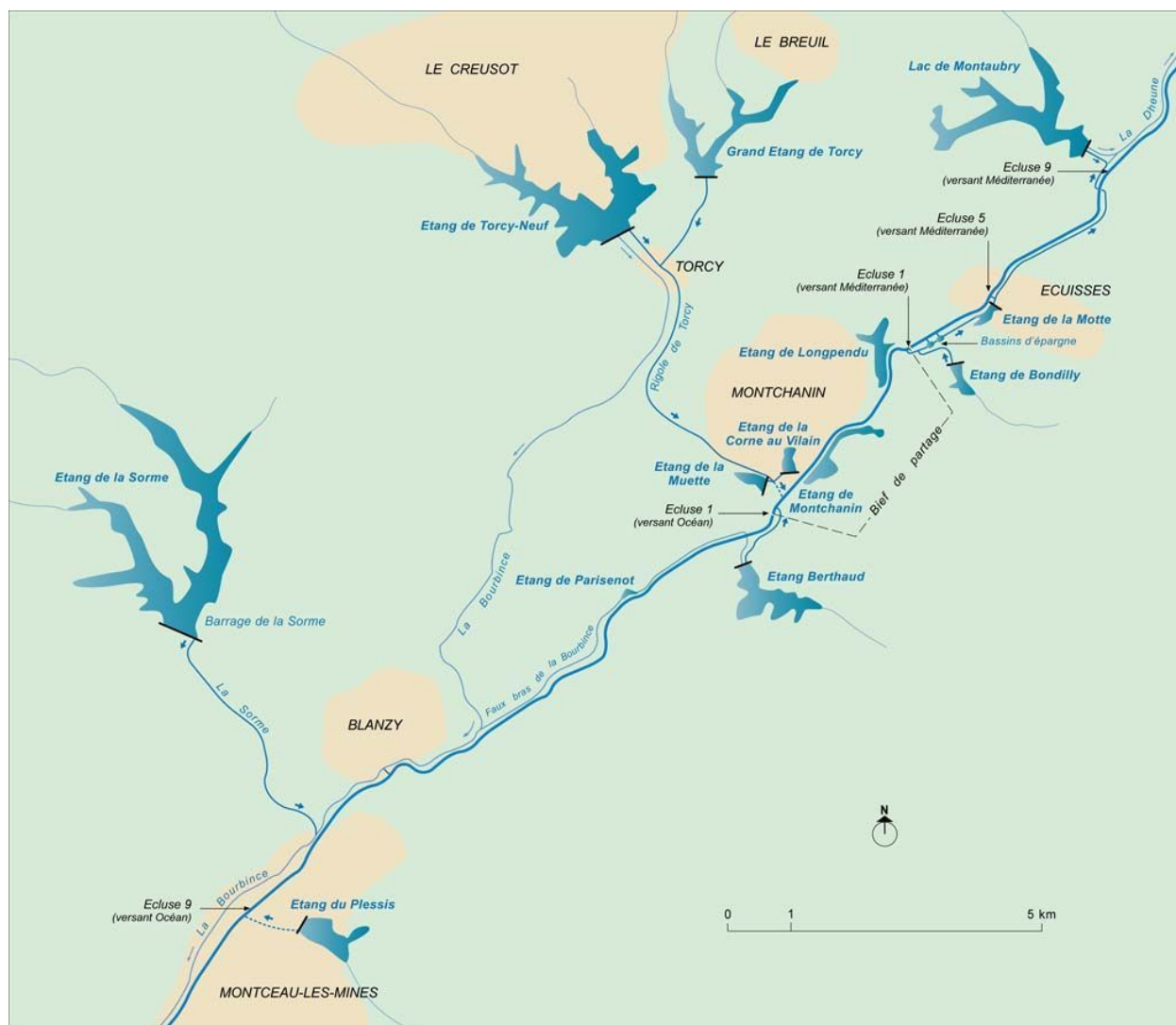
Carte schématique de l'ensemble des réservoirs concourant à l'alimentation du canal du Centre au niveau du bief de partage.
