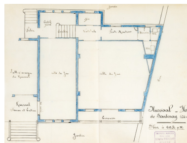
Plan de distribution des deux salles de jeux du casino. Phot. Pierre-Marie Barbe- Richaud, Autr. Pierrot IVR43_20192100118NUC2P
