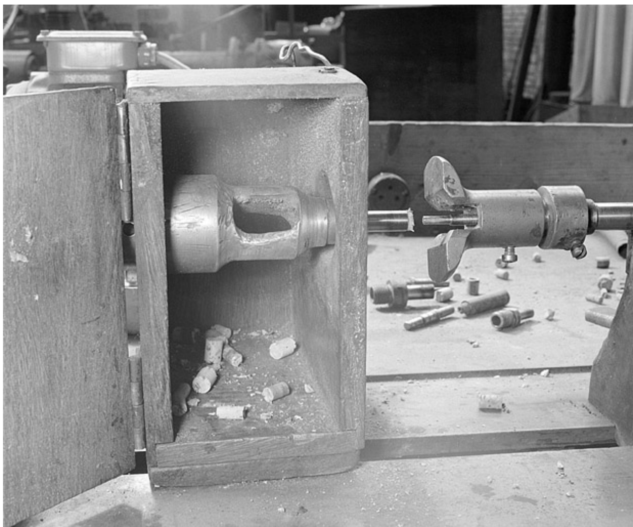
Détail de l'outil de coupe.
