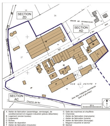
Plan-masse et de situation. Assemblages d'extraits de plans cadastraux numérisés, sections AC, AD, ZD, le tout réduit à 1:1700. Source : Direction générale des Finances Publiques - Cadastre ; mise à jour : 2008. Dess. André Céréza IVR43_20087000473NUDA
