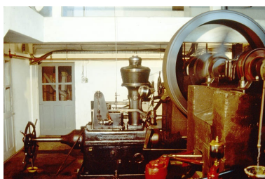
Bâtiment d'eau : régulateur S.A.C.M.
