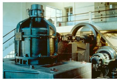
Bâtiment d'eau : réducteur Messian et dynamo de la Cie Générale Electrique.
