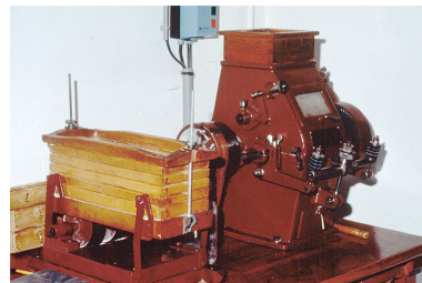
Atelier de fabrication (L), 1er étage : appareil à cylindres et plansichter du laboratoire. Phot. Laurent Poupard IVR43_19893900599ZA
