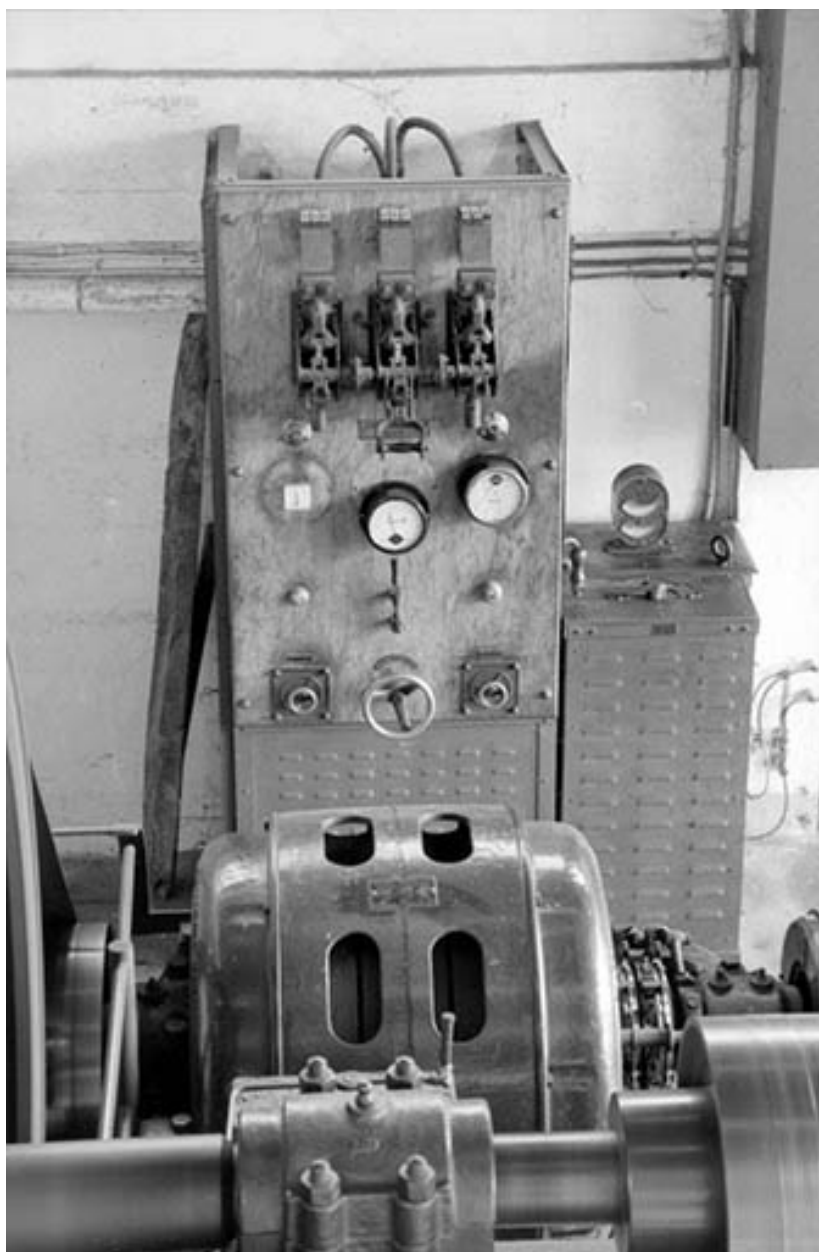
Bâtiment d'eau : tableau de commande électrique.
