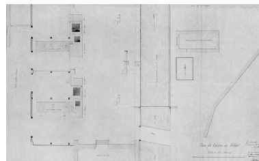
Plan de l'usine de Belfort (Haut-Rhin) [plan de détail]. Phot. Jérôme Mongreville IVR43_20019000025V
