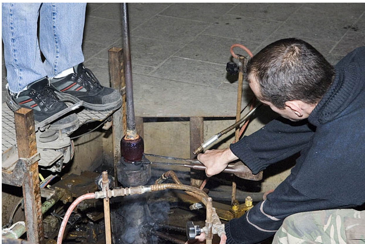
Soufflage. Détail du poste de moulage (ou "gamin mécanique").
