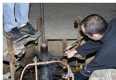
Soufflage. Détail du poste de moulage (ou "gamin mécanique"). Phot. Jérôme Mongreville IVR43_20077000897NUCA
