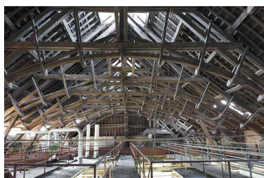
Atelier des fours. Vue du comble depuis la croupe nord. Phot. Jérôme Mongreville IVR43_20077000932NUCA
