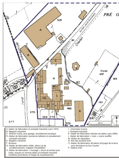
Plan-masse de l'usine. Extrait du plan cadastral numérisé, 2008, section B, 1:2500 agrandi à 1:2000. Source : Direction générale des Finances Publiques - Cadastre ; mise à jour : 2008.
