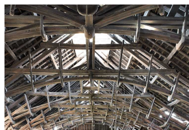
Charpente de l'atelier des fours. Détail des assemblages par étriers. Phot. Jérôme Mongreville IVR43_20077000933NUCA
