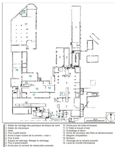
Plan-masse de la verrerie en 1991. Dess. André Céréza IVR43_20087001048NUDA
