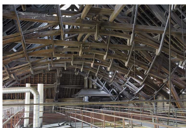
Charpente de l'atelier des fours. Détail des fermes. Phot. Jérôme Mongreville IVR43_20077000931NUCA
