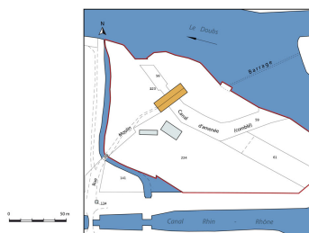
Plan-masse et de situation. Dess. Mathias Papigny IVR43_20132502658NUDA
