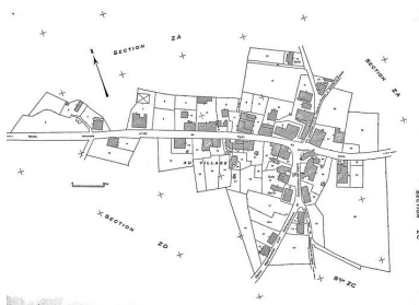
Plan cadastral, 1968, section AB, échelle 1 : 1000. Phot. Yves Sancey IVR43_19852500018V
