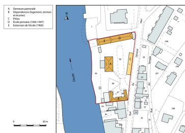
Plan-masse et de situation. Extrait du plan cadastral numérisé, section AO, échelle 1:1000. Dess. Mathias Papigny IVR43_20142500584NUDA
