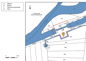
Plan masse et de situation. Dess. Mathias Papigny IVR43_20177000360NUDA
