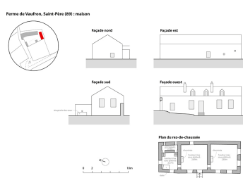
Relevé de la maison : plan et élévations, 1/200. Dess. Aline Thomas IVR26_20268900253NUDA
