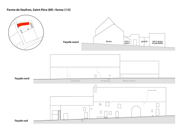
Relevé de la ferme (1/3) : élévations, 1/200. Dess. Aline Thomas IVR26_20268900254NUDA
