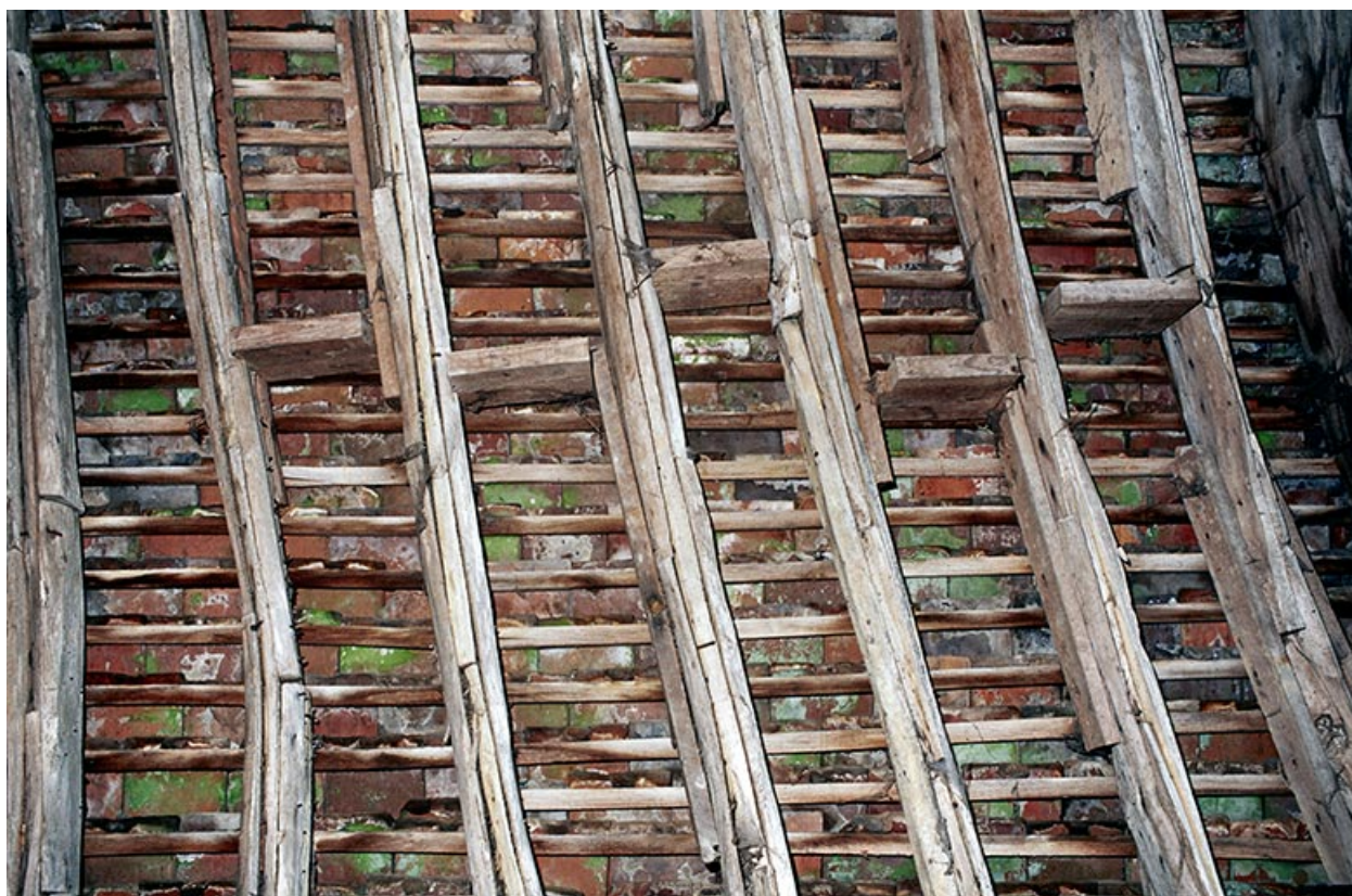
Charpente du séchoir, détail en 2002.
