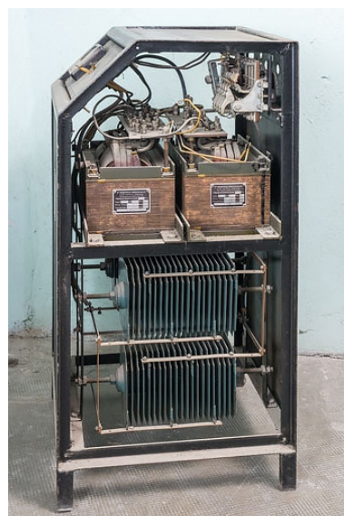
Redresseur Rectarc désaffecté : vue de profil, tôle de protection enlevée. Phot. Pierre-Marie Barbe-Richaud IVR26_20222100056NUC4A
