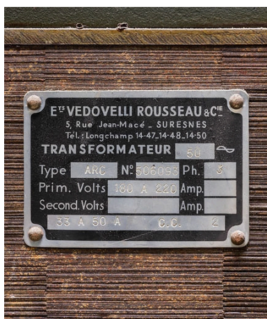
Redresseur Rectarc désaffecté : plaque de constructeur sur l'un des éléments. Phot. Pierre-Marie Barbe-Richaud IVR26_20222100064NUC2A
