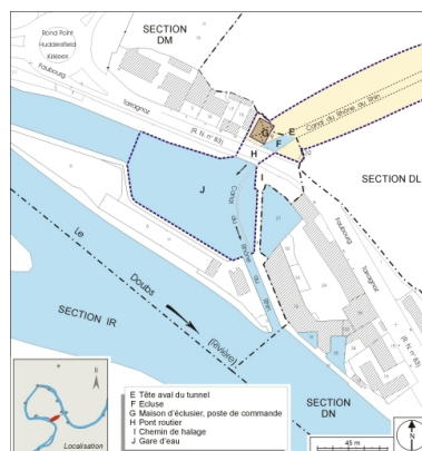
Plan-masse et de situation de la partie aval. Dess. André Céréza IVR43_20062500340NUDA
