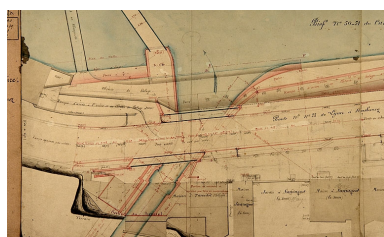
Dérivation sous la citadelle de Besançon [...] Dessins du pont sous la route nationale n° 83 à Tarragnoz [plan], 1877. Phot. Yves Sancey, Phot. Rascol IVR43_20062500125NUCA
