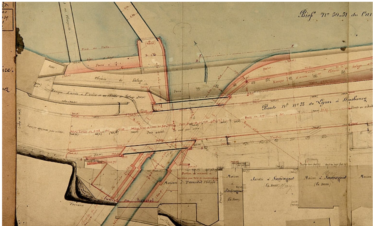
Dérivation sous la citadelle de Besançon [...] Dessins du pont sous la route nationale n° 83 à Tarragnoz [plan], 1877.
