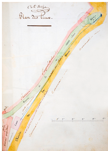
Plan des lieux [pour la construction de la fontaine-lavoir de la Sauce à Sceaux-sur-Saône-et-Saint-Albin]. 1848. Repro. Jérôme Mongreville, Autr. Noirot-Hugon IVR43_20197000038NUC4A
