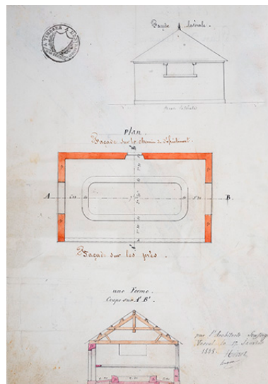
Plan et coupe transversale [pour la construction de la fontaine-lavoir de la Sauce à Sceaux-sur-Saône-et-Saint-Albin]. 1848. Repro. Jérôme Mongreville, Autr. Noirot-Hugon IVR43_20197000039NUC4A
