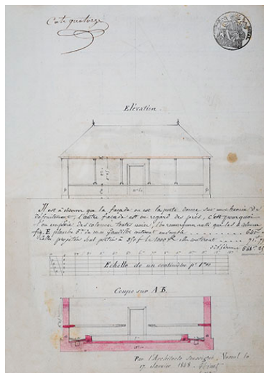
Élévation et coupe longitudinale [pour la construction de la fontaine-lavoir de la Sauce à Sceaux-sur-Saône-et-Saint-Albin]. 1848. Repro. Jérôme Mongreville, Autr. Noirot-Hugon IVR43_20197000040NUC4A
