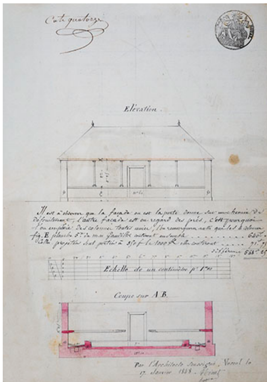
Élévation et coupe longitudinale [pour la construction de la fontaine-lavoir de la Sauce à Sceaux-sur-Saône-et-Saint-Albin]. 1848.
