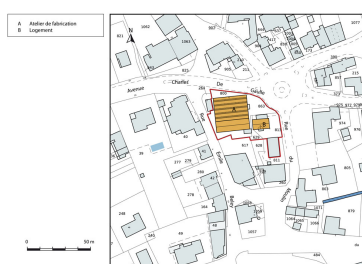
Plan-masse et de situation. Dess. Mathias Papigny IVR43_20132502588NUDA
