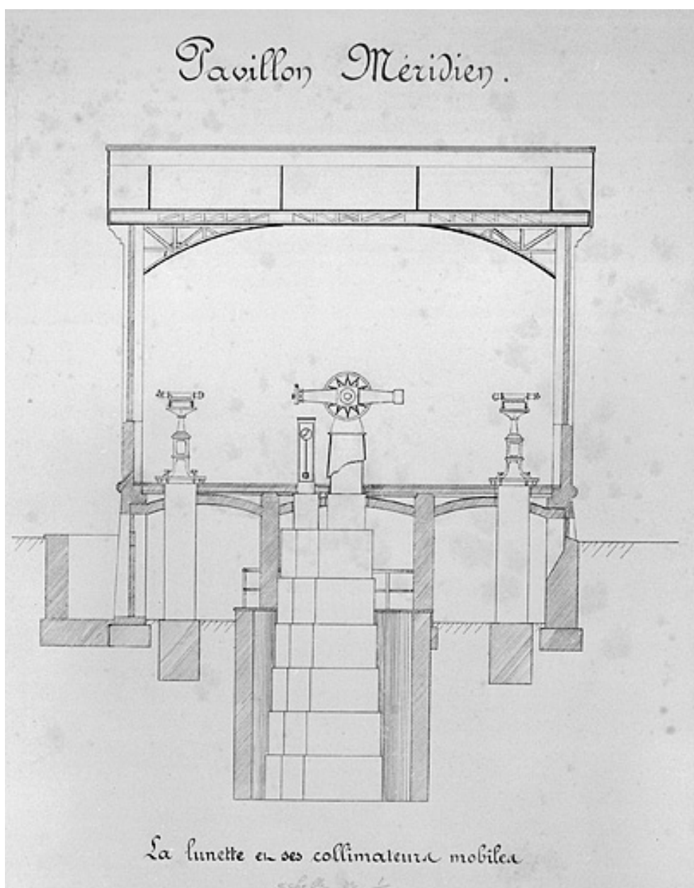
Pavillon méridien. La lunette et ses collimateurs mobiles [coupe nord-sud], limite 19e siècle 20e siècle.
