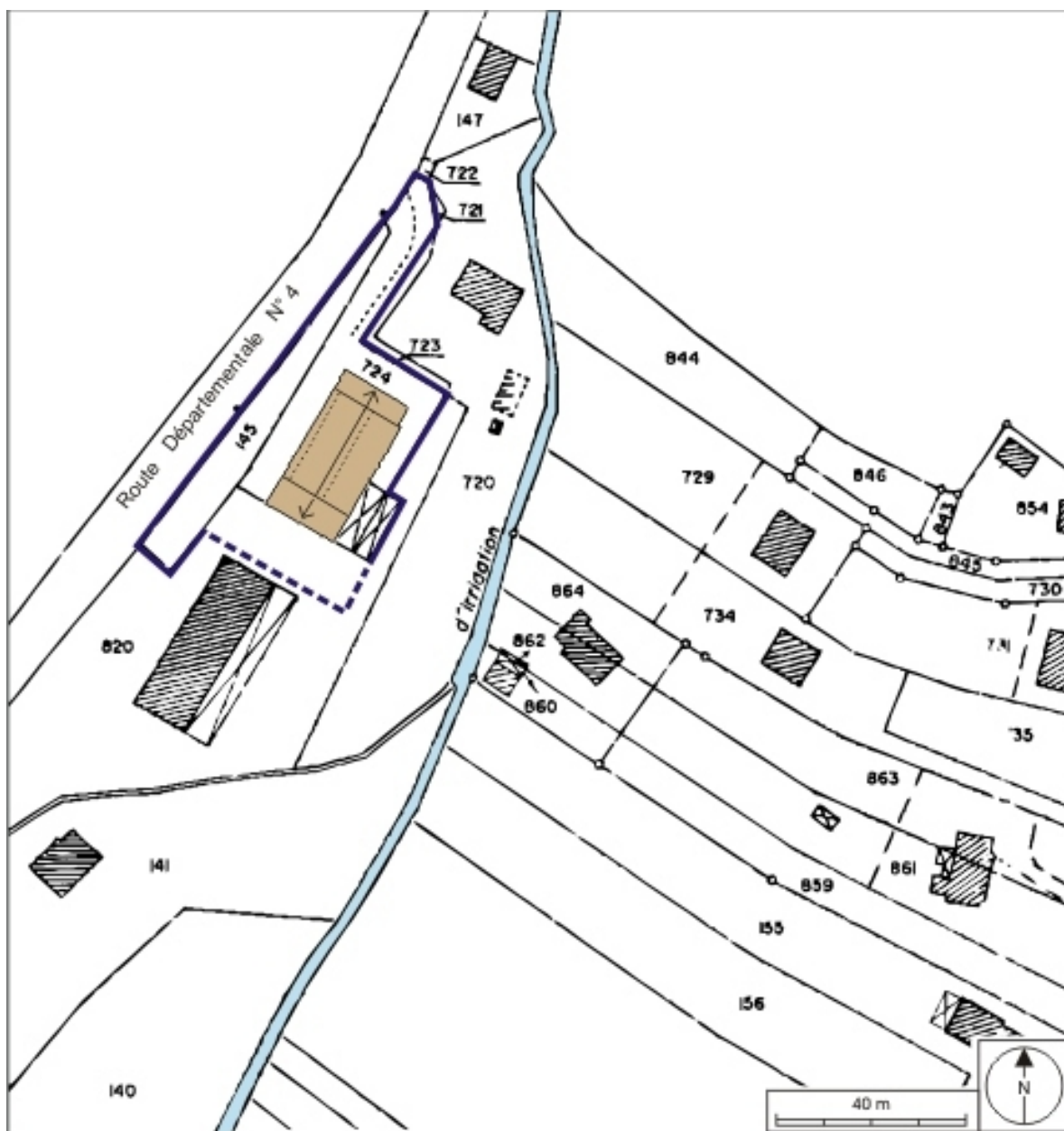
Plan-masse et de situation. Extrait du plan cadastral numérisé, 2008, section G, échelle 1:1250. Source : Direction générale des Finances Publiques - Cadastre ; mise à jour : 2008.
