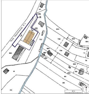
Plan-masse et de situation. Extrait du plan cadastral numérisé, 2008, section G, échelle 1:1250. Source : Direction générale des Finances Publiques - Cadastre ; mise à jour : 2008. Dess. André Céréza IVR43_20087000176NUDA
